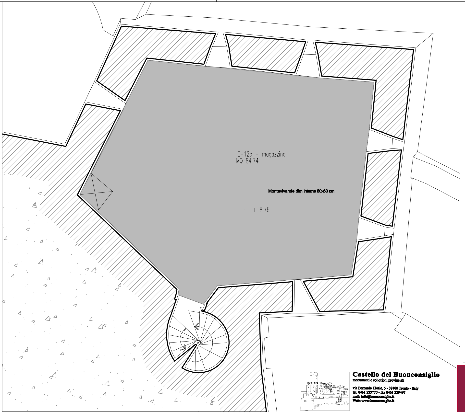
PIANTA MAGAZZINO 1:50
